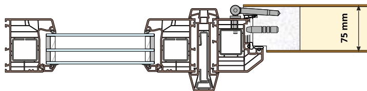
Sujungimo skerspjūvis varčia su langeliu ARCTIC PLUS
