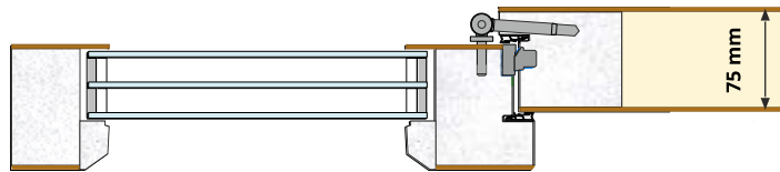
Sujungimo skerspjūvis varčia su langeliu VISION
