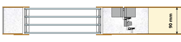
Sujungimo skerspjūvis varčia su langeliu ULTIMATE
