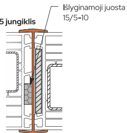
Jungiklių schema naudojama linijose
